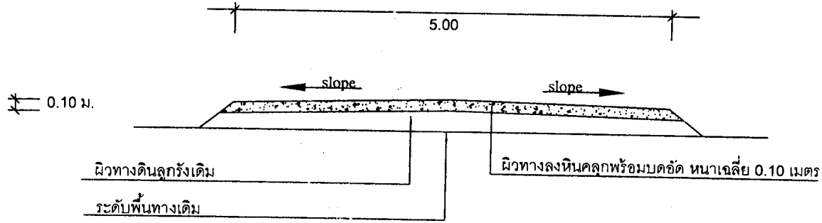
รูปตัด ก - ก ซอยทรายทอง 1-2 Not to Scale
