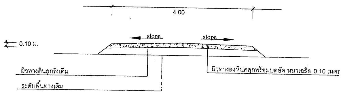
รูปตัด ก - ก ซอยสะเตางาม Not to Scale
