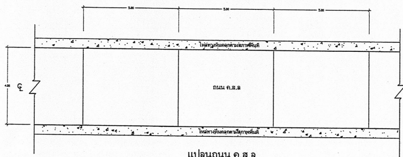
แปลนถนน ค.ส.ล. Scale 1:100
