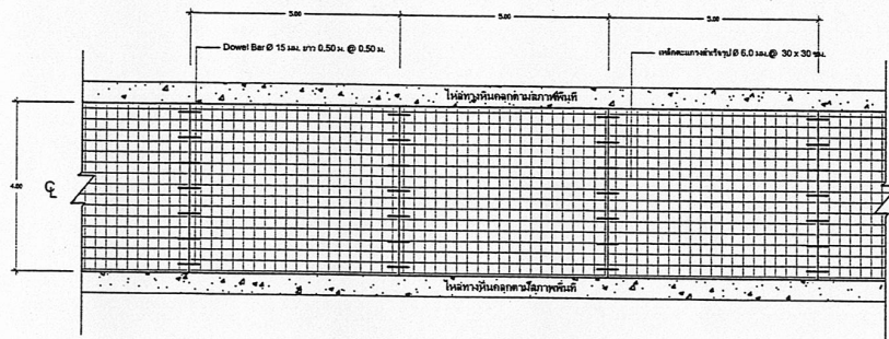
แปลนแสดงการเสริมเหล็กถนน ค.ส.ล. Scale 1:100
