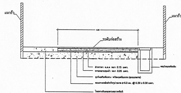
รูปตัดตามขวางถนน ค.ส.ล. scale 1:50
