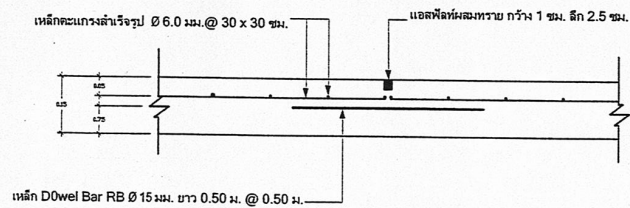
ขยายรอยต่อ CONTRACTION JOINT Scale 1:10
